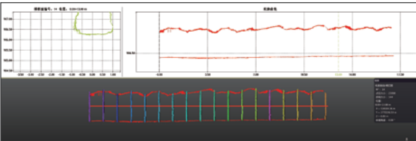
巷道断面分析
